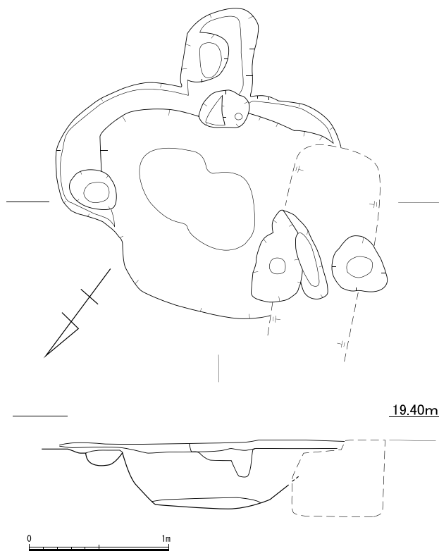
第7図 SK01実測図 (1/40)
