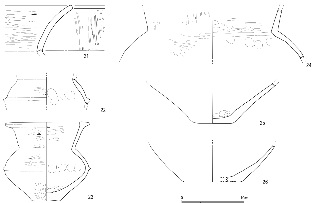
第10図 包含層出土遺物実測図①
