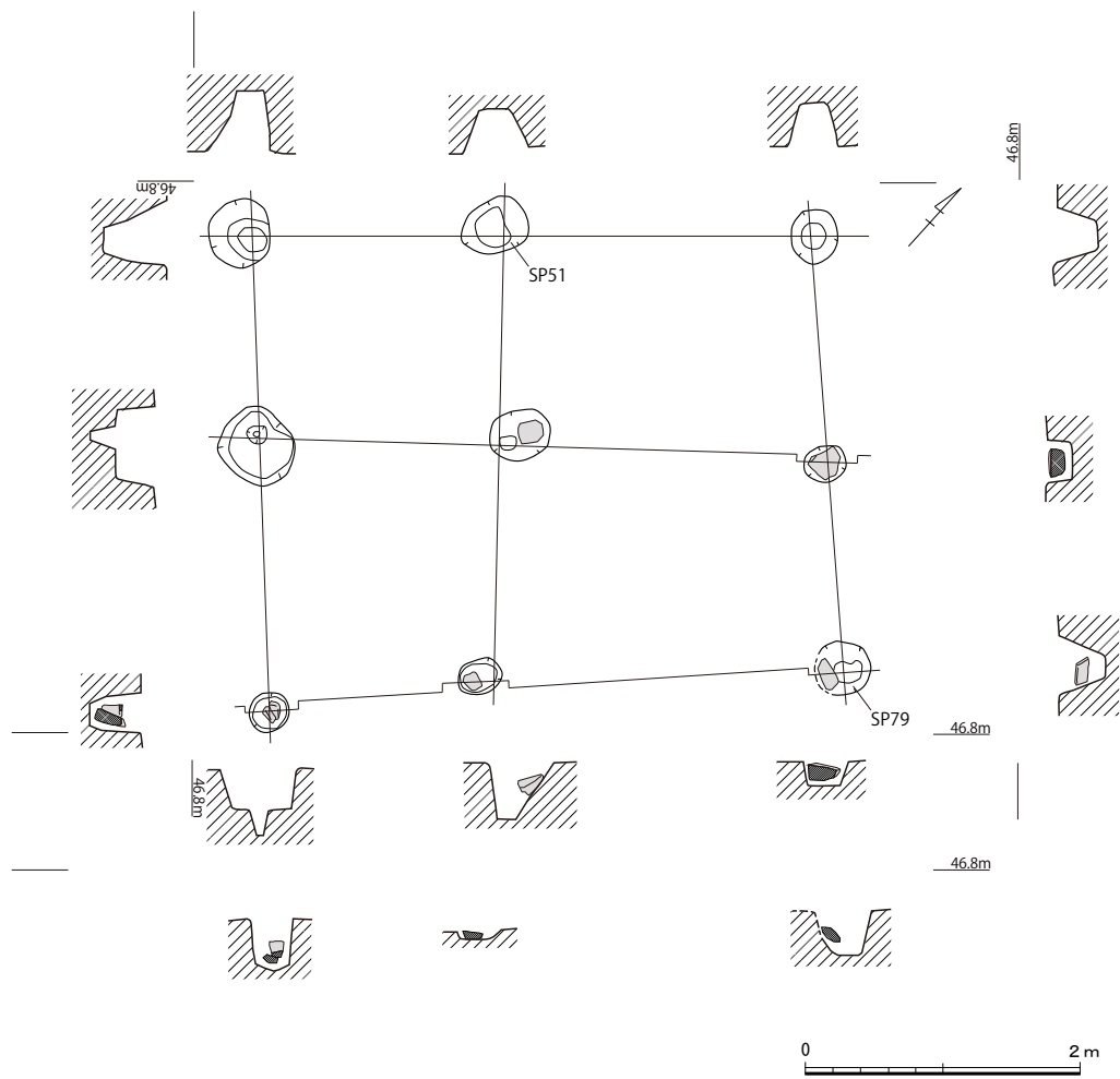
第5図 SB01 実測図 (1/60)
