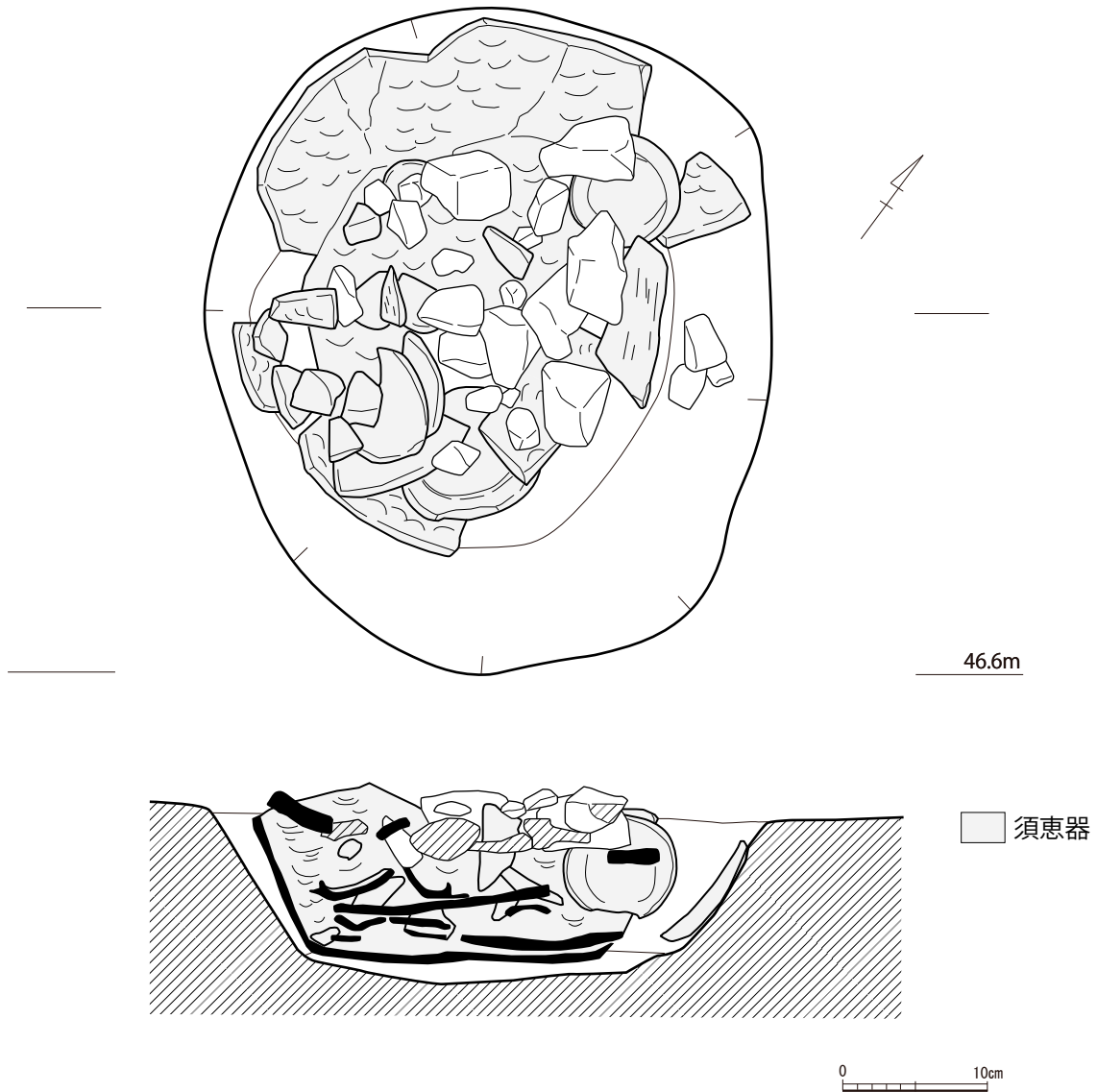
第7図 SX02 実測図 (1/5)
