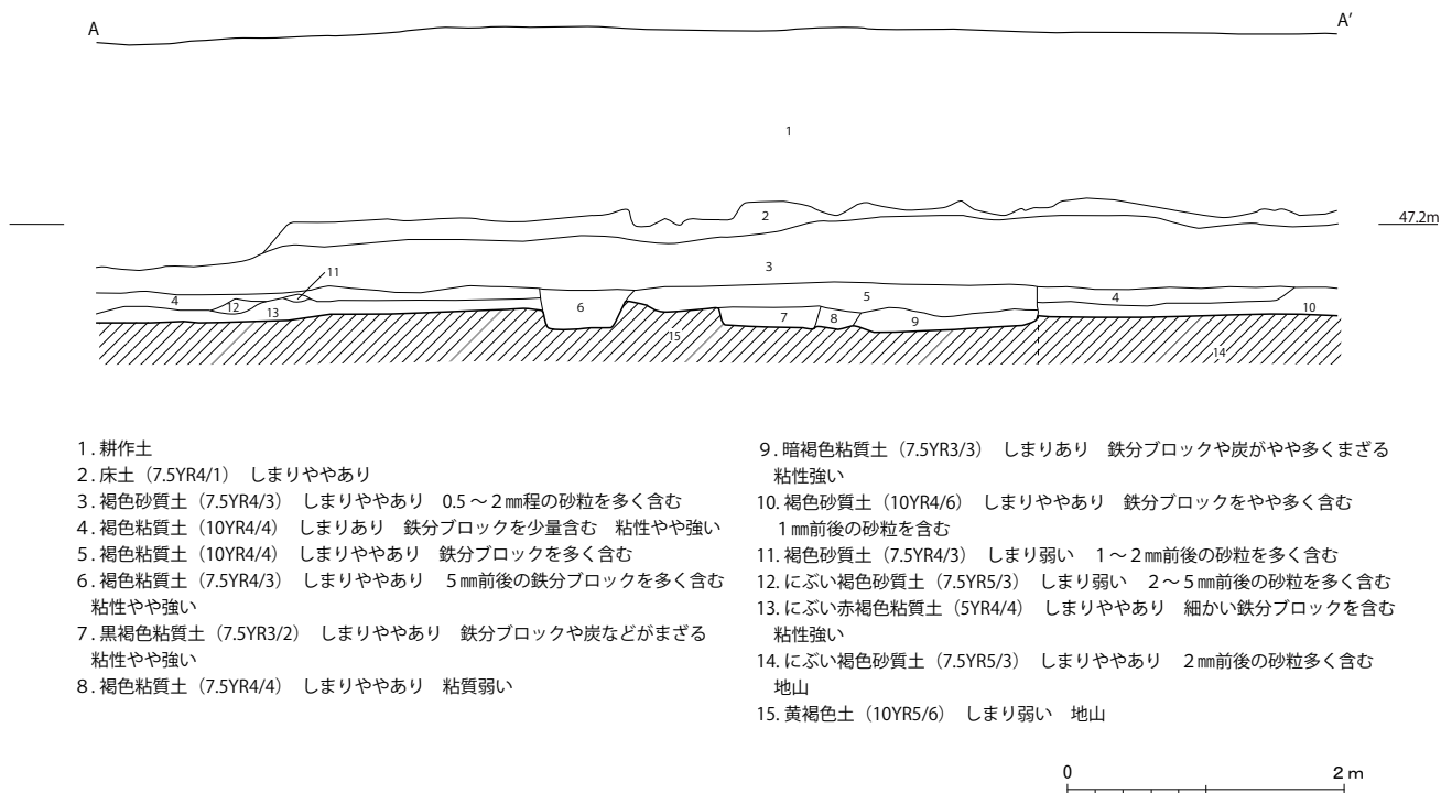
第4図 調査区南壁面土層実測図 (1/60)
