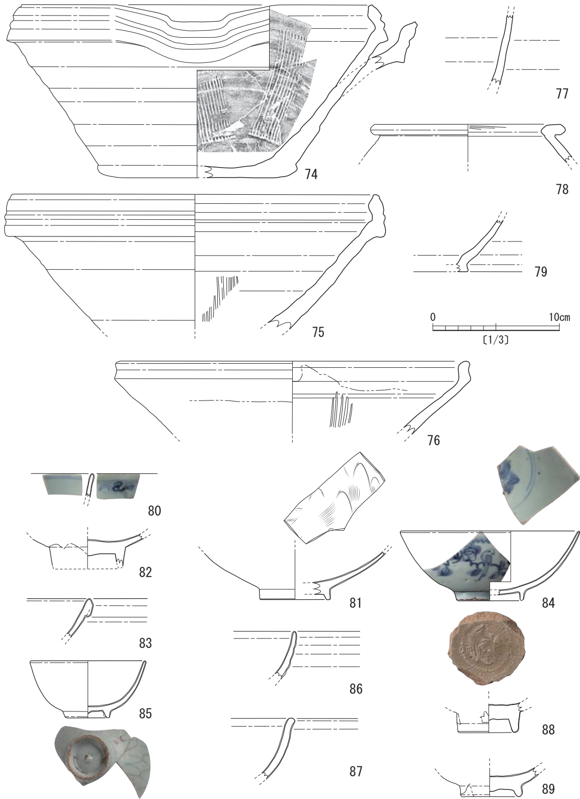
第12図 第4次調査 SK02出土遺物実測図② (S=1/3)
