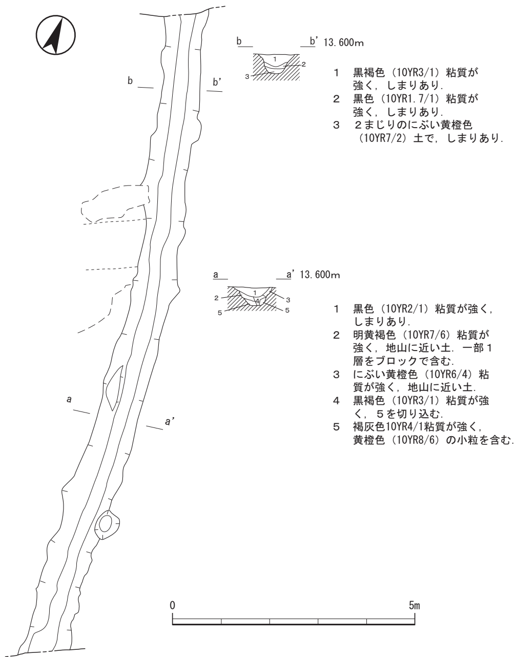
第18図 第7次調査 SD01実測図 (S=1/80)
