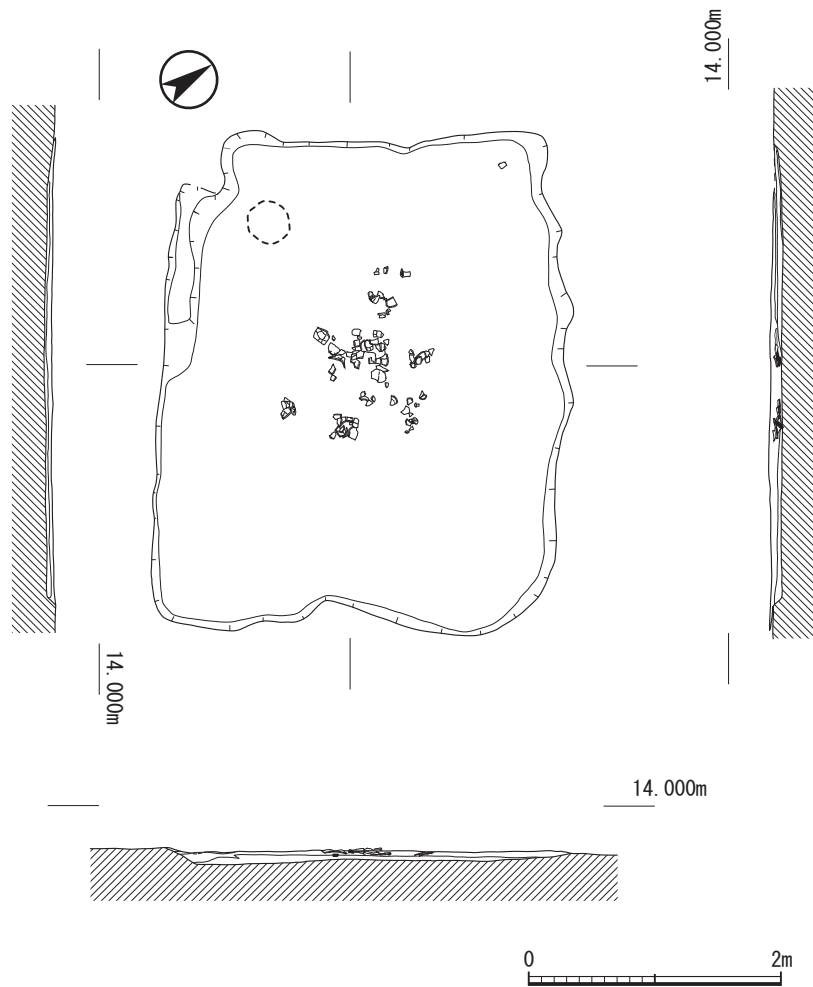
第21図 第7次調査 SX03実測図 (S=1/60)
