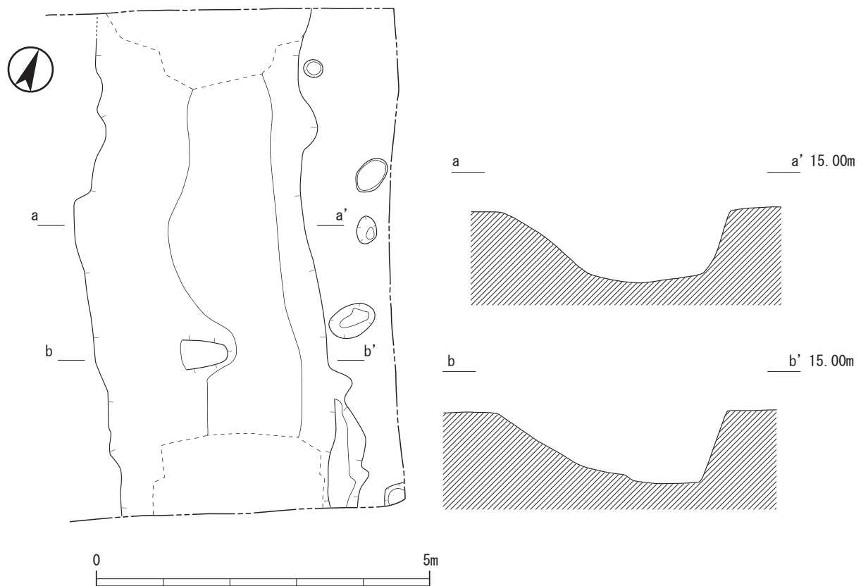
第4図 第4次調査 SD01実測図 (S=1/80)
