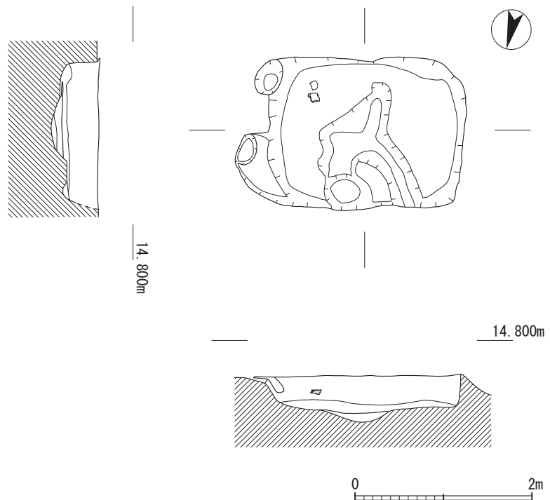
第8図 第4次調査 SK01実測図 (S=1/60)
