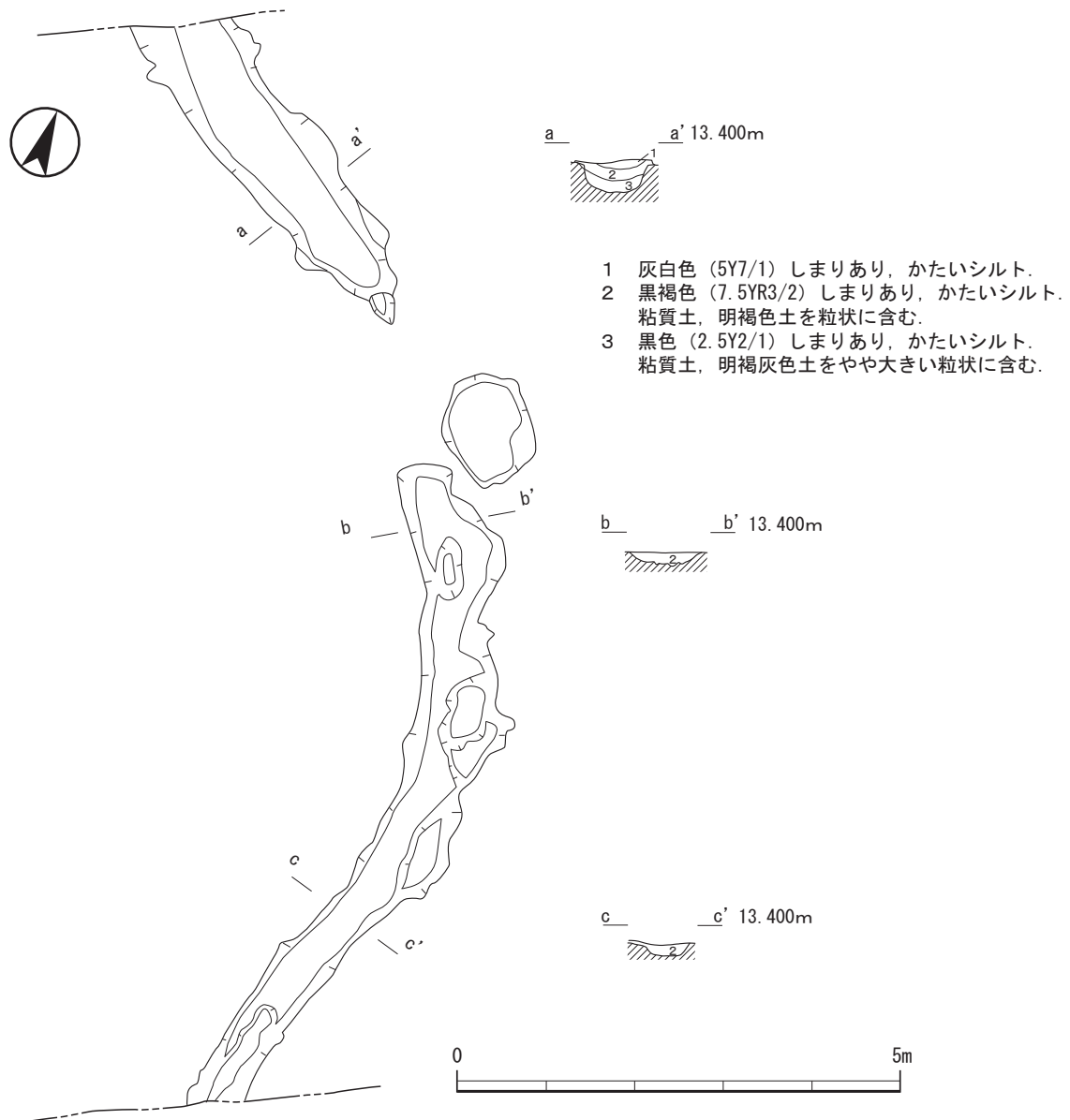
第20図 第7次調査 SD02実測図 (S=1/80)
