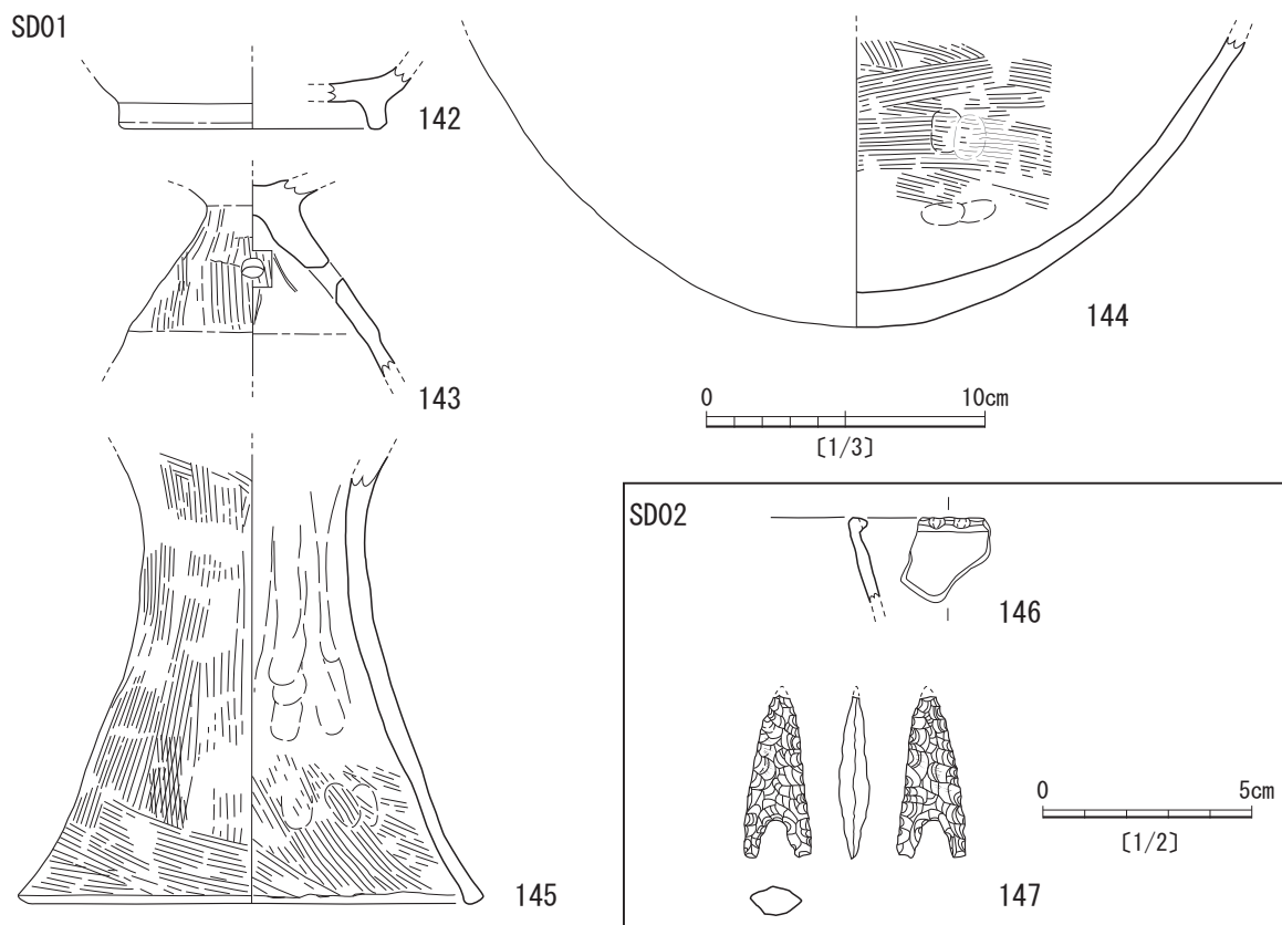
第19図 第7次調査 SD01・SD02出土遺物実測図 (147はS=1/2、その他はS=1/3)
